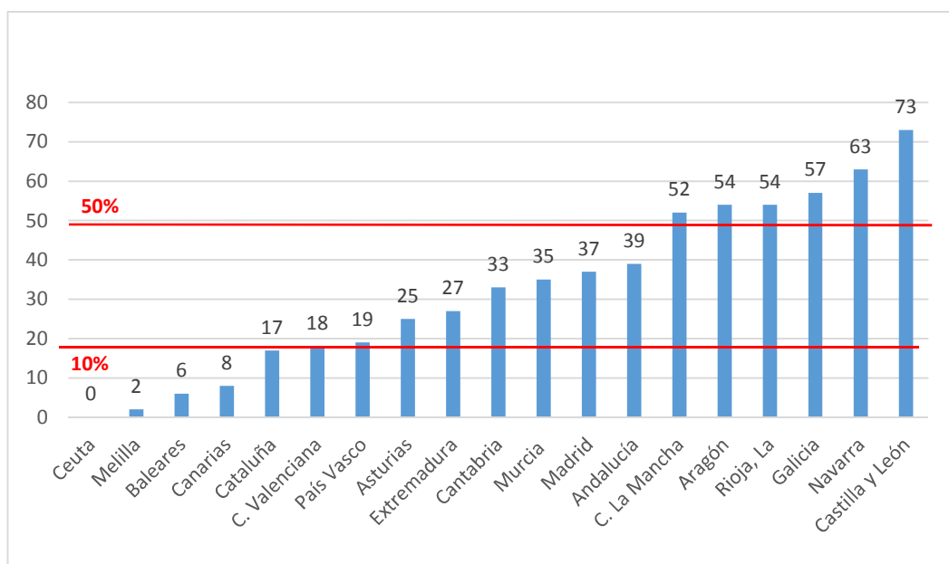
Gráfico 14. Generación renovable por CCAA en %
