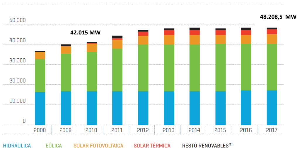
Gráfico 41. Evolución de la potencia instalada renovable.
