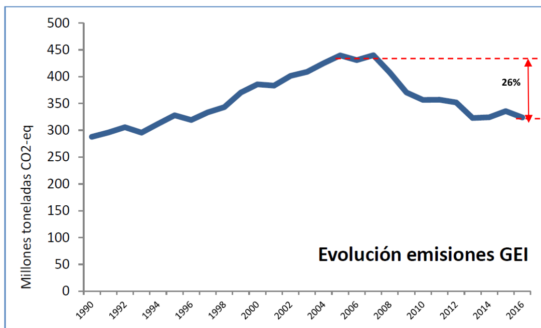
Gráfico 4. Emisiones de GEI España 1990-2016
