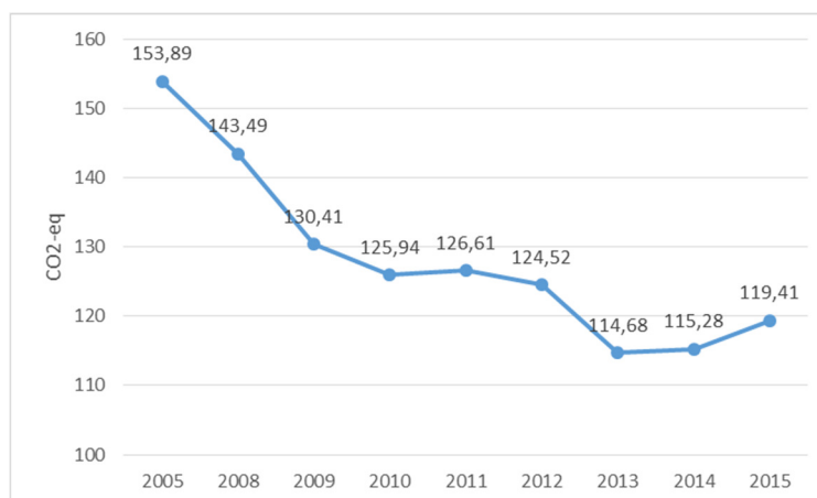
Gráfico 23. Emisiones de GEI (CO2 equivalente) Índice 1990=100
